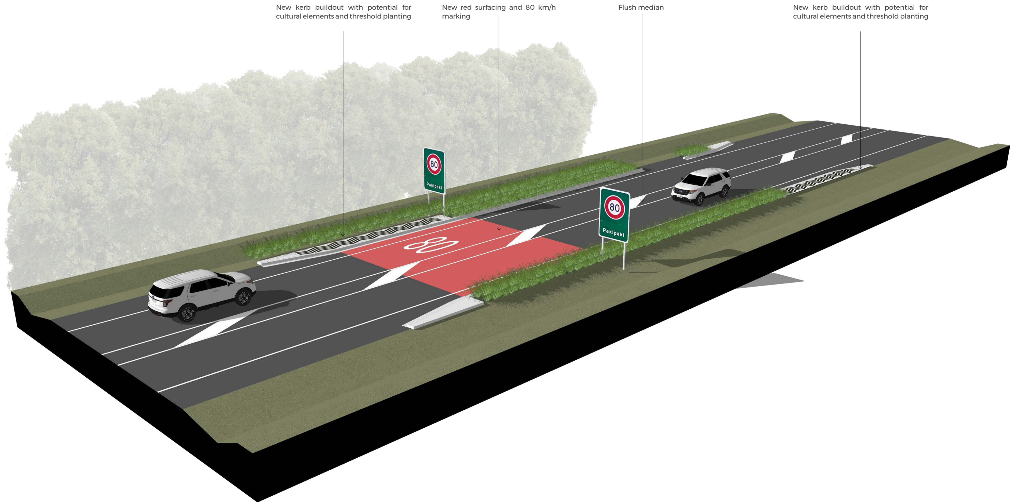
Zone A: Perspective
